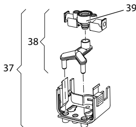
Abb. 23: Milcheinheit ausbauen
