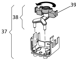
Abb. 21: Einlauf drehen
