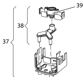
Fig. 23: Smontaggio del gruppo latte
