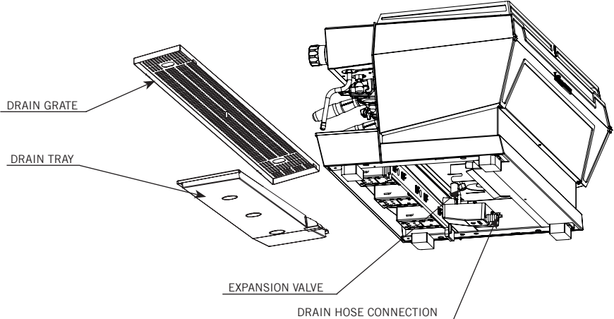
Fig. 3 - Installation Nomenclature
