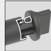
easyclean valdiklis – tinkamos padėties nustatymas (kaiščiiai išėmoje)
