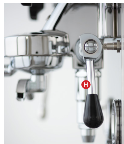
Fig H. Levier d'infusion entièrement orienté vers le bas, l'eau ne s'écoule pas et la pompe est éteinte (Position « Off »)
