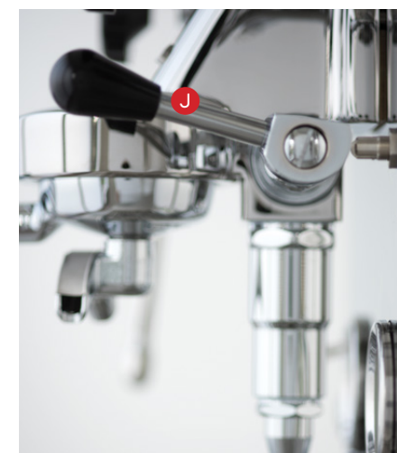
Fig J. Levier d'infusion orienté vers le haut et eau chauffée qui s'écoule
